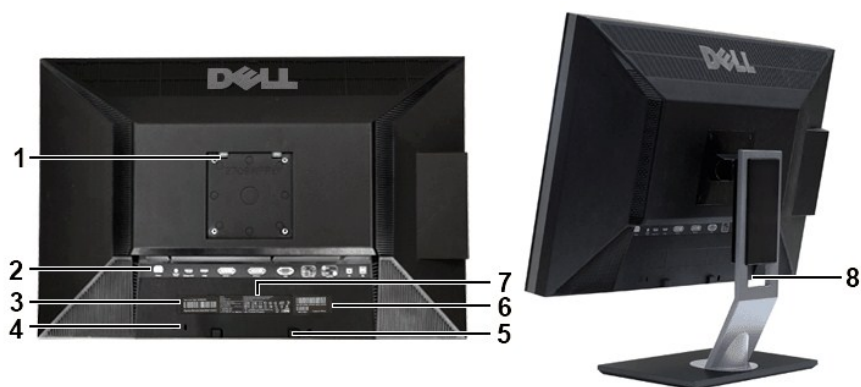
背面図
